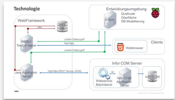
Abb.: WebFramework / Technischer Überblick
